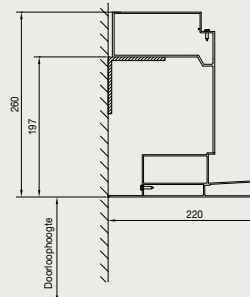
Pivot Fassadenmontage
