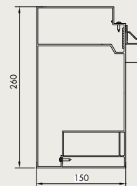
Span Fassadenmontage
