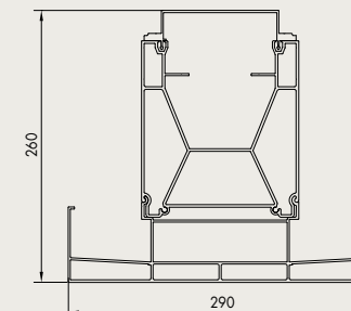
Pivot gekoppelt
