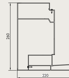
Pivot Fassadenmontage
