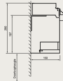
Span Fassadenmontage
