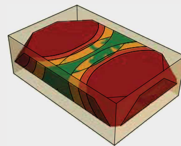
Wärmeeffekt mit 2 Seiten beheizt (Format 6 x 4 m)
